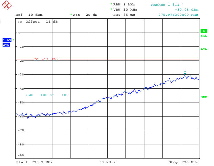
Band13 GSM UL Left Side Pre AGC+10dB
