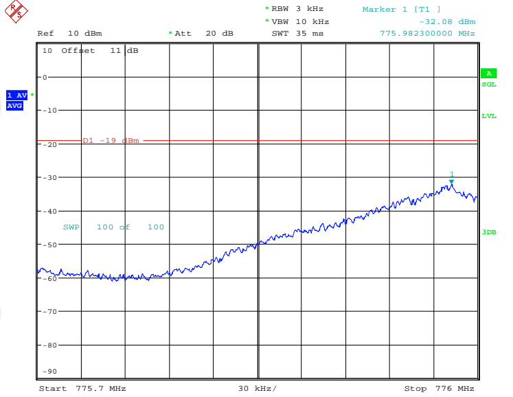
Band13 GSM UL Left Side Pre AGC
