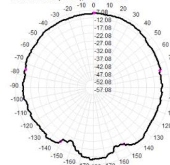
1960.0MHz Total(E2-YZ), Max= -9.04dBi
