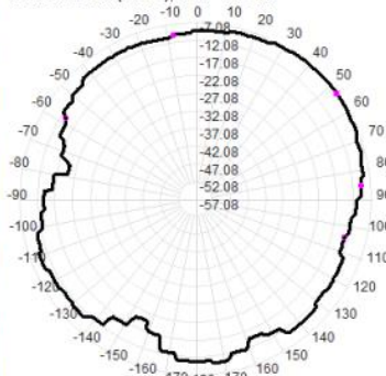
1960.0MHz Total(E1-XZ), Max= -7.08dBi
