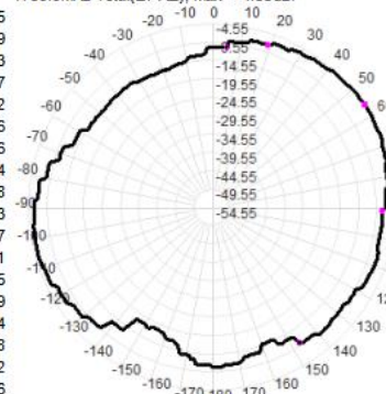
1750.0MHz Total(E1-XZ), Max= -4.55dBi
