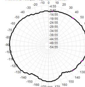
1750.0MHz Total(E2-YZ), Max= -5.63dBi
