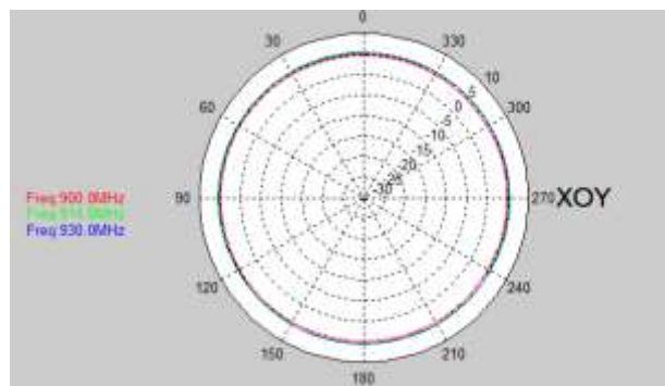
E-plane
