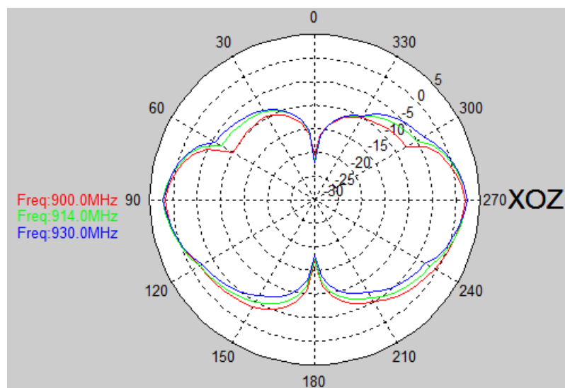
E-plane
