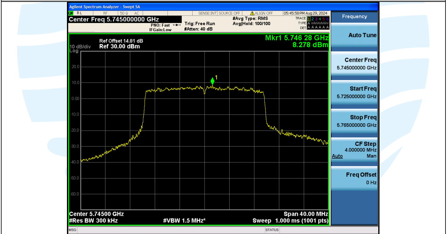
11AX20MIMO-Ant1-5785-PASS
