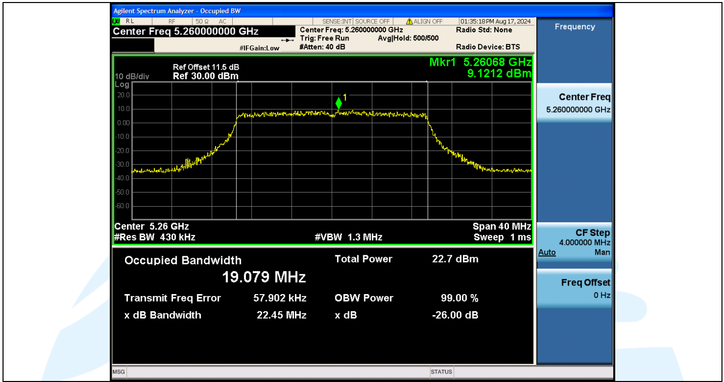
11AX20MIMO-Ant2-5260
