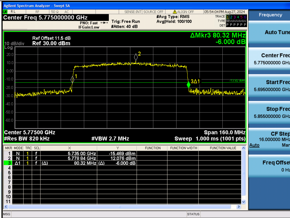
11AX80MIMO-Ant3-5775
