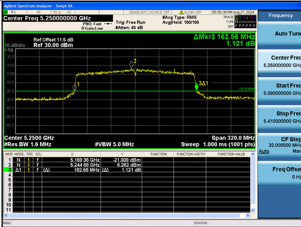
11AX160MIMO-Ant3-5250
