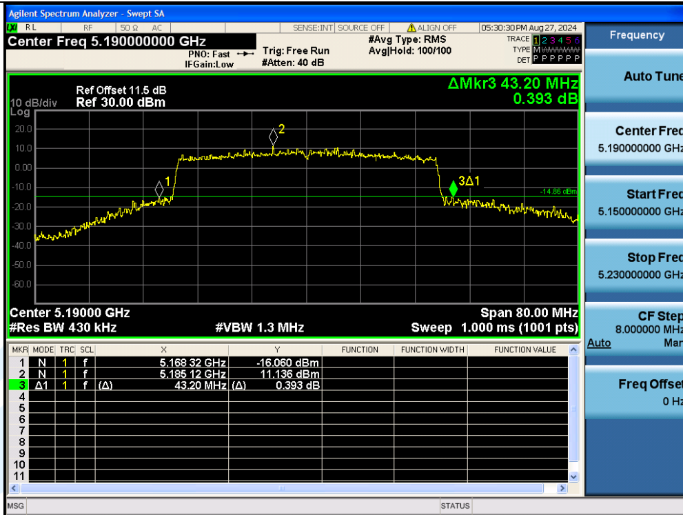
11AX40MIMO-Ant3-5190
