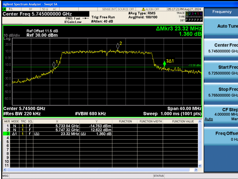
11AX20MIMO-Ant3-5745
