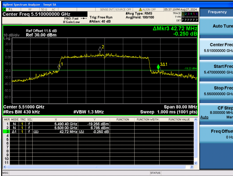
11AX40MIMO-Ant3-5510
