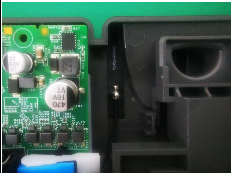
2.4G Antenna
