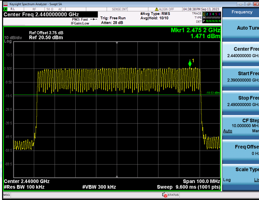
2 Band Edge (Hopping) NVNT ANT1 1-DH5 Hopping
