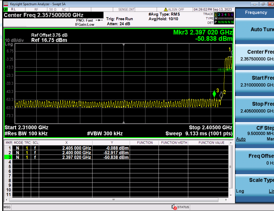
2 Band Edge (Hopping) NVNT ANT1 1-DH5 Hopping
