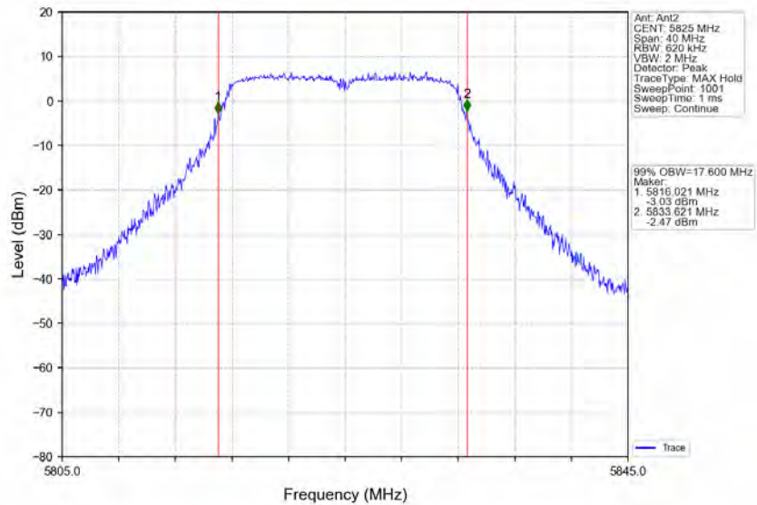
802.11a_HCH_5825MHz_Ant2_NTNV
