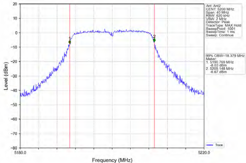
802.11n(HT20)_MCH_5200MHz_Ant2_NTNV
