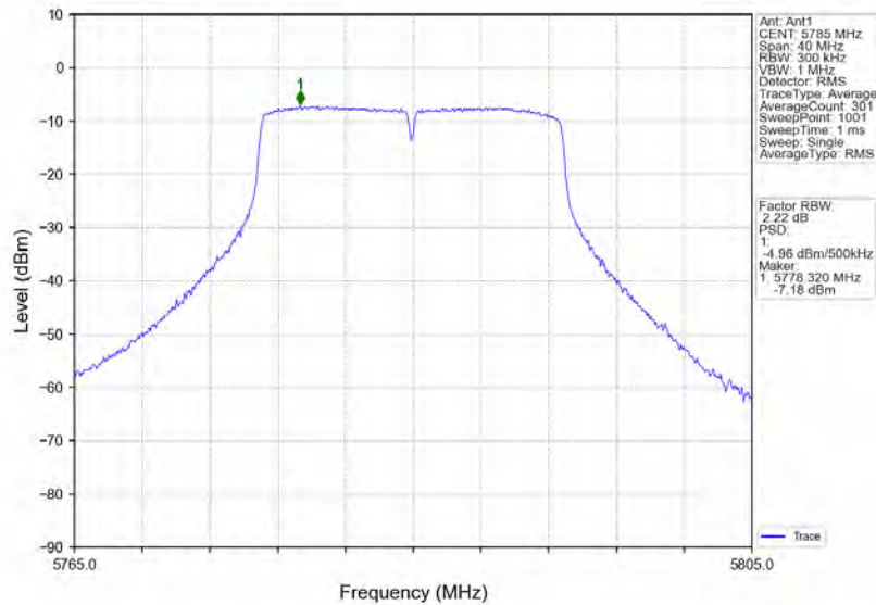
802.11n(HT20)_MCH_5785MHz_Ant1_NTNV
