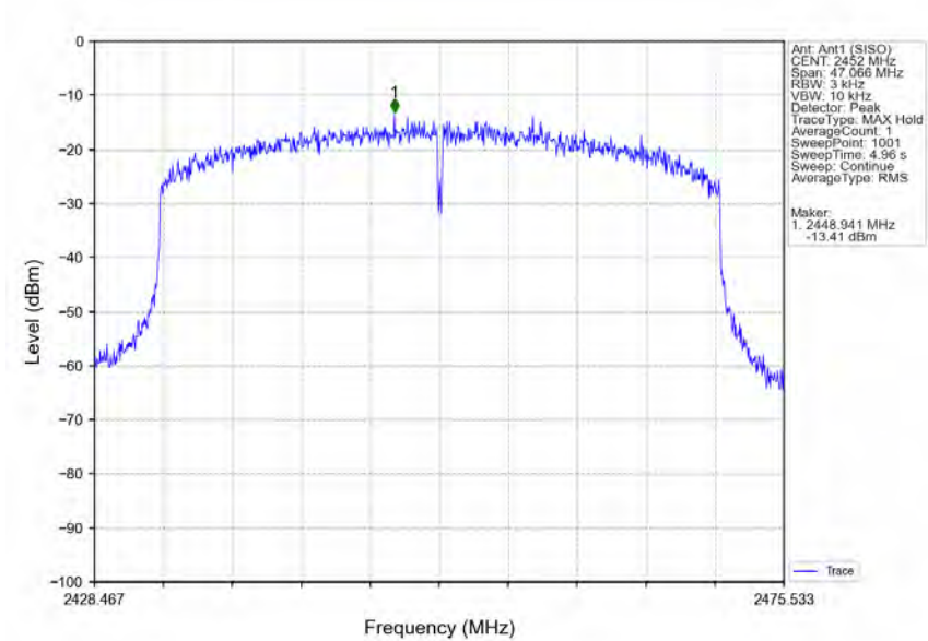
802.11ax(HEW40) HCH 2452MHz RU484 Left Ant1 (SISO) NTNv
