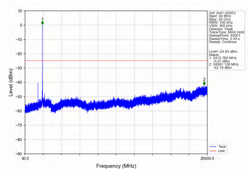
802.11ax(HEW20) LCH_2412MHz_RU242_Left_Ant1 (SISO) NTN
