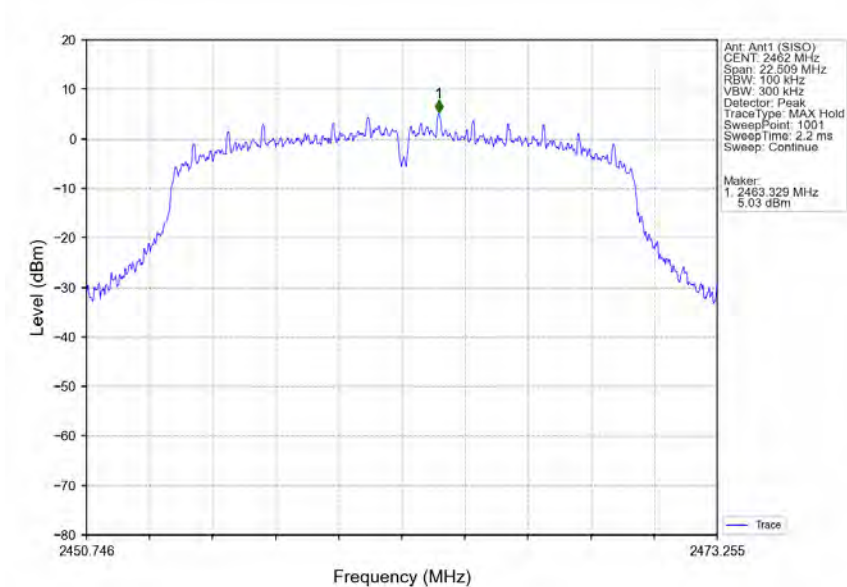
802.11g_HCH_2462MHz_Ant1 (SISO)_NTNV
