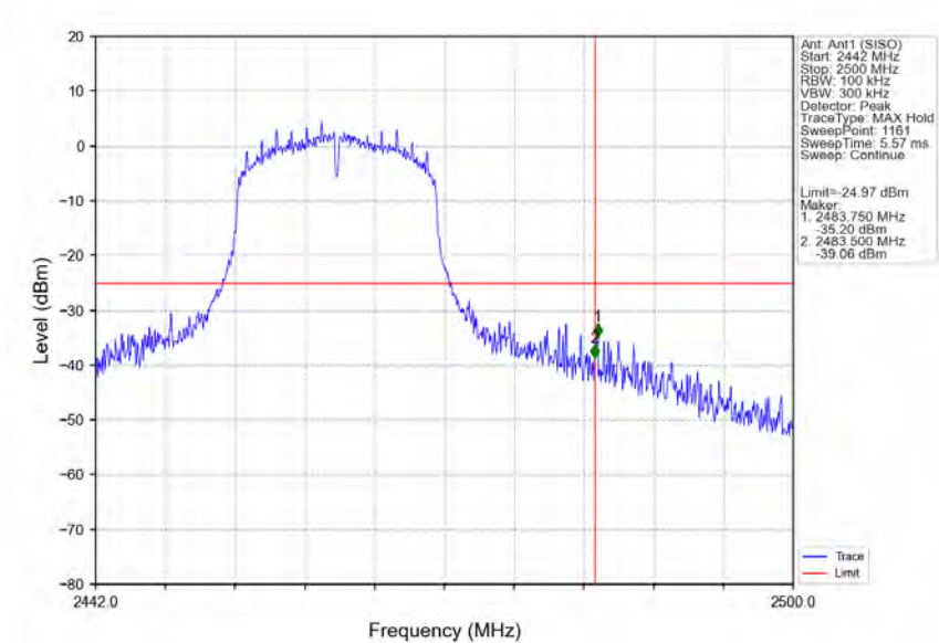
802.11g_HCH_2462MHz_Ant1 (SISO)_NTNV
