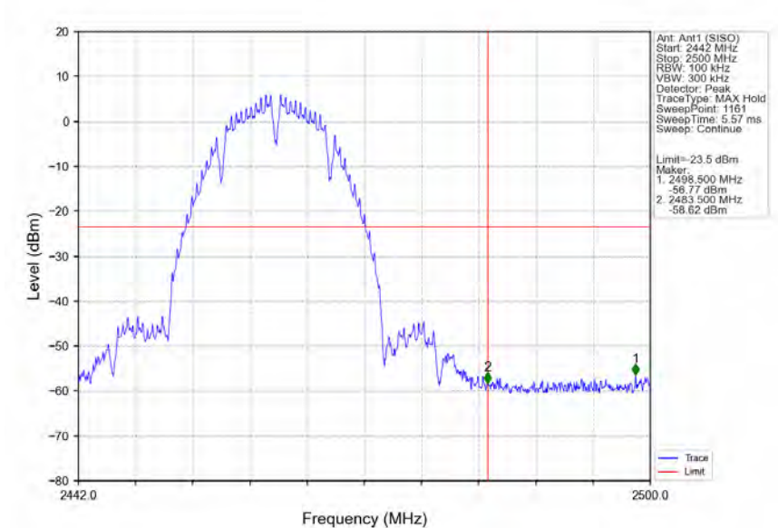
802.11b HCH 2462MHz Ant1 (SISO) NTVN
