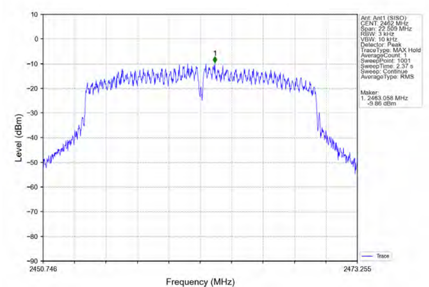
802.11g_HCH_2462MHz_Ant1 (SISO)_NTNV
