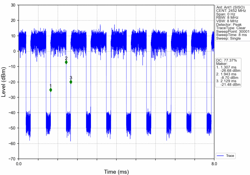
802.11n(HT40)_HCH_2452MHz_Ant1 (SISO)_NTNV
