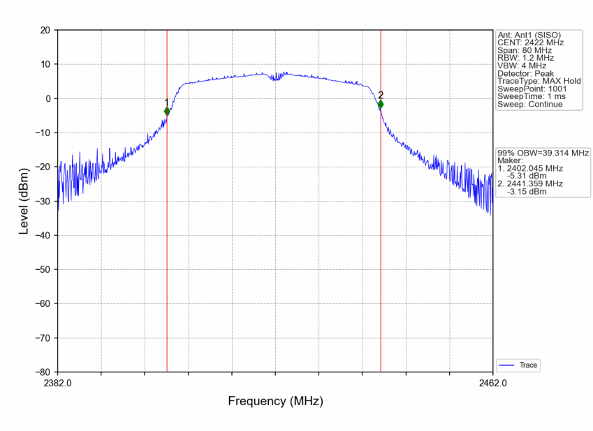
802.11n(HT40)_LCH_2422MHz_Ant1 (SISO)_NTNV
