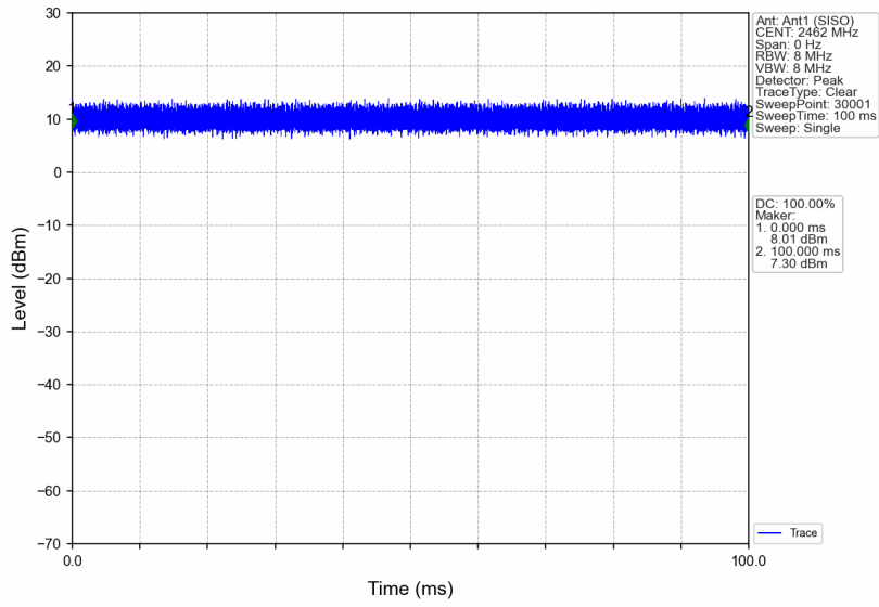
802.11n(HT20)_HCH_2462MHz_Ant1 (SISO)_NTNV
