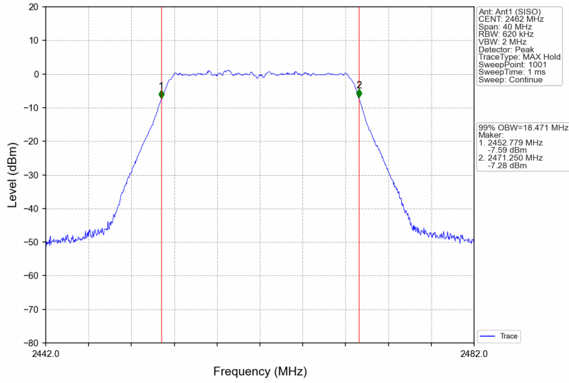
802.11n(HT20)_HCH_2462MHz_Ant1 (SISO)_NTNV
