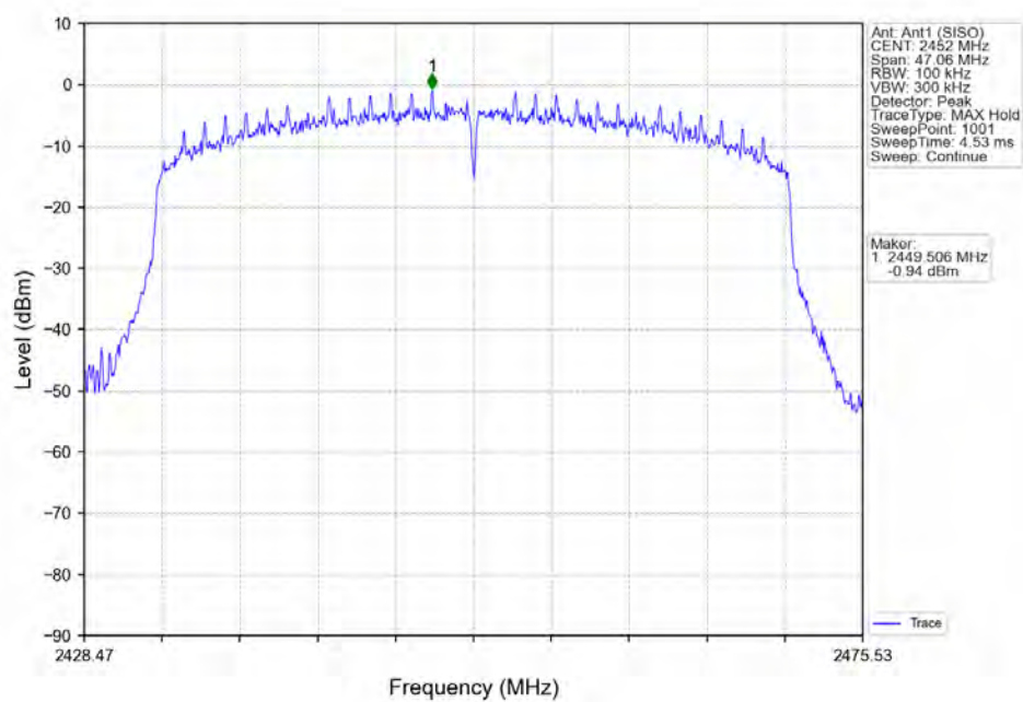
802.11ax(HEW40)_HCH_2452MHz_RU484_Left_Ant1 (SISO)_NTNV
