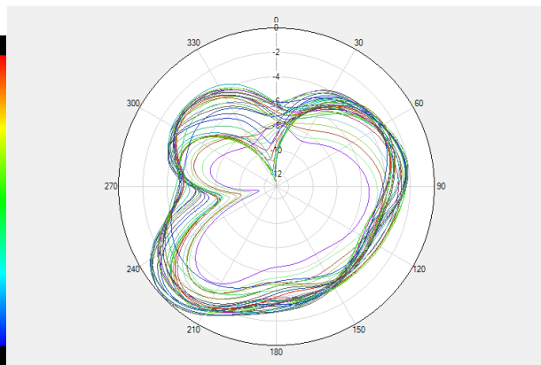
THETA=90 2D
