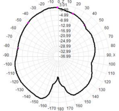
2450.0MHz Total(E1-XZ), Max= 1.01dBi
