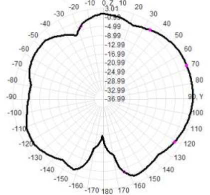
2450.0MHz Total(E2-YZ), Max= 2.92dBi
