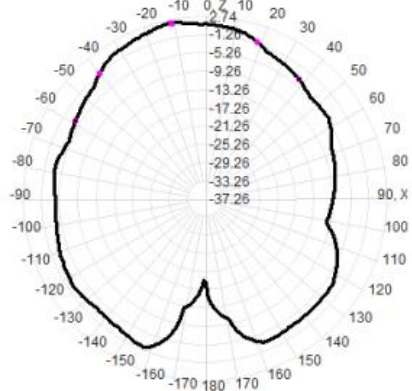
2500.0MHz Total(E1-XZ), Max= 1.99dBi
