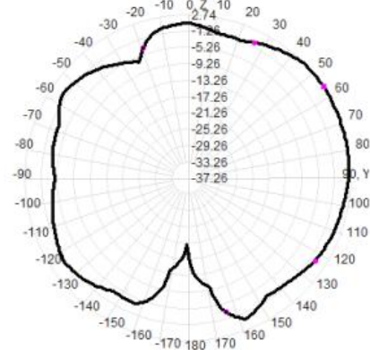
2500.0MHz Total(E2-YZ), Max= 2.74dBi
