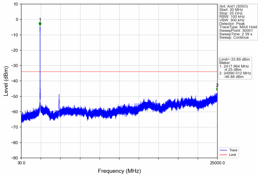
802.11n(HT40) MCH 2437MHz Ant1 (SISO) NTV
