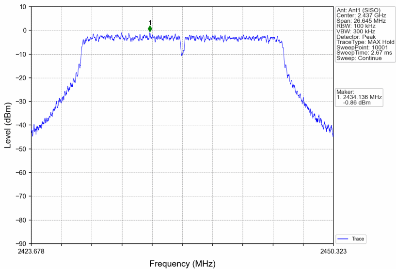
802.11n(HT20) MCH 2437MHz Ant1 (SISO) NTV
