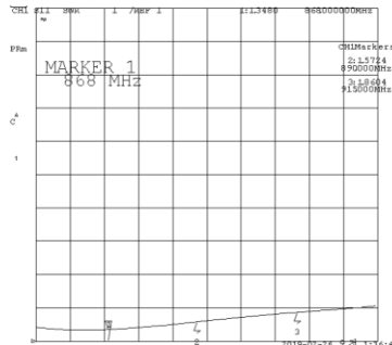
VSWR
