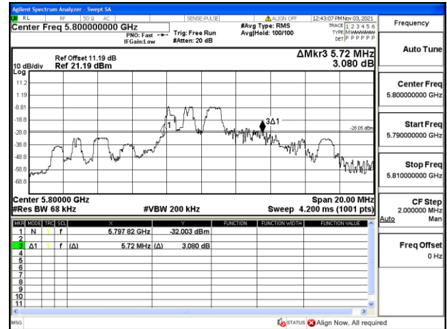
5800MHz
