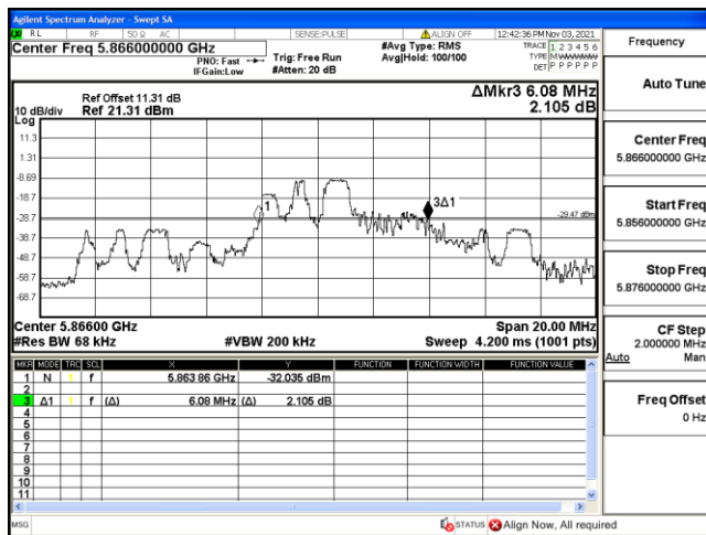
5866MHz
