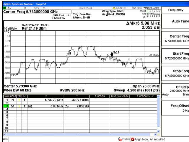
5733MHz
