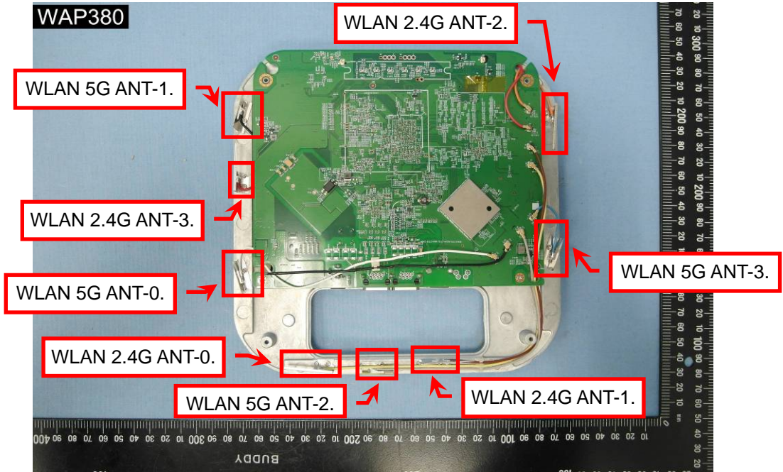
EUT Photo (12)
