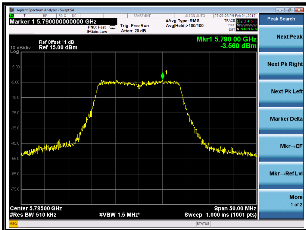
(Channel 157: 5785MHz @ 802.11ac)
