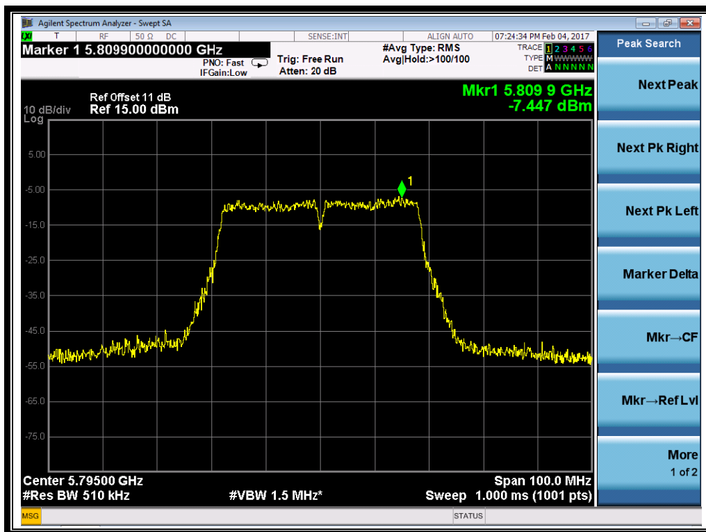
(Channel 159: 5795MHz @ 802.11ac)
