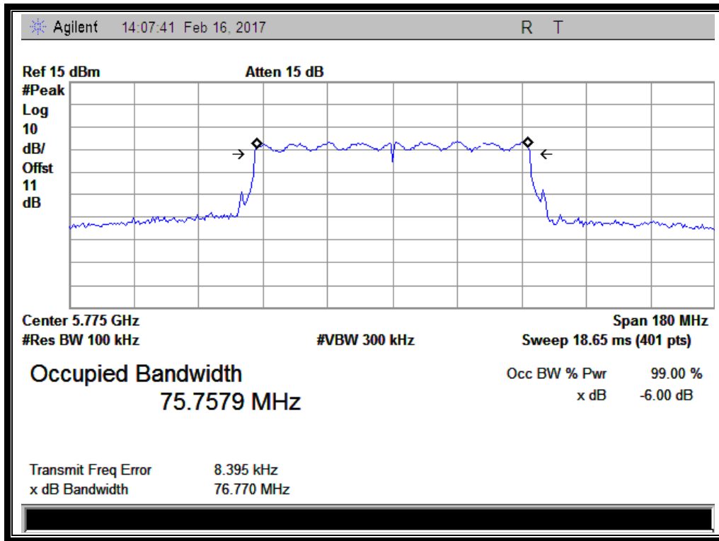
(Channel 155: 5775MHz @ 802.11ac)
