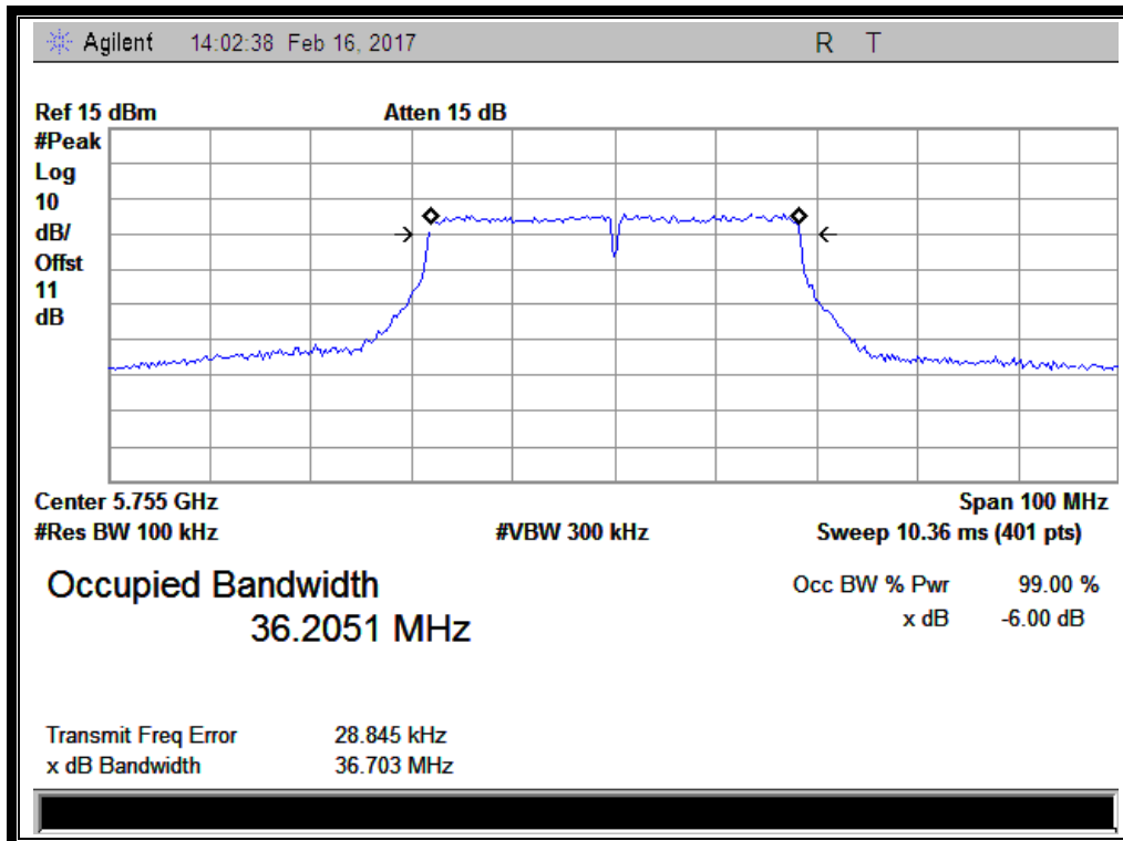
(Channel 151: 5755MHz @ 802.11ac)
