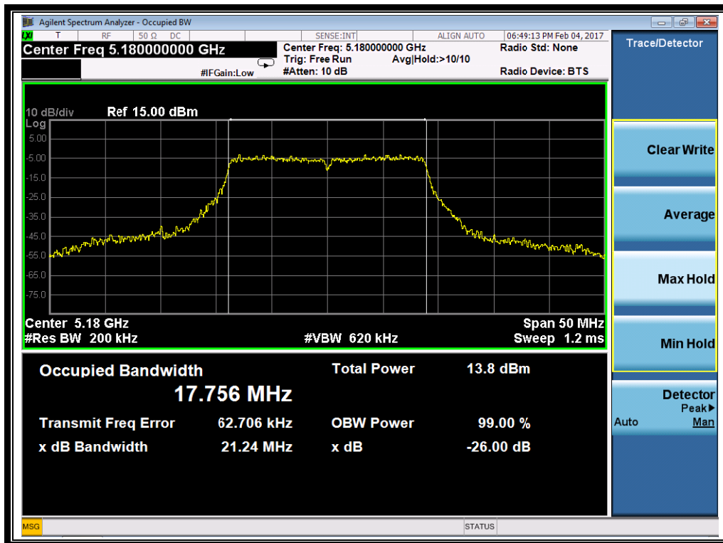
(Channel 36: 5180MHz @ 802.11ac)
