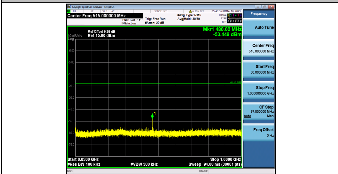
11N40SISO_Ant0_2452_30~1000
