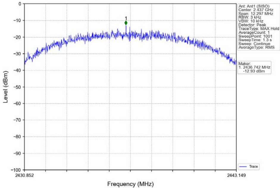
802.11b_MCH_2437MHz_Ant1 (SISO)_NTNV
