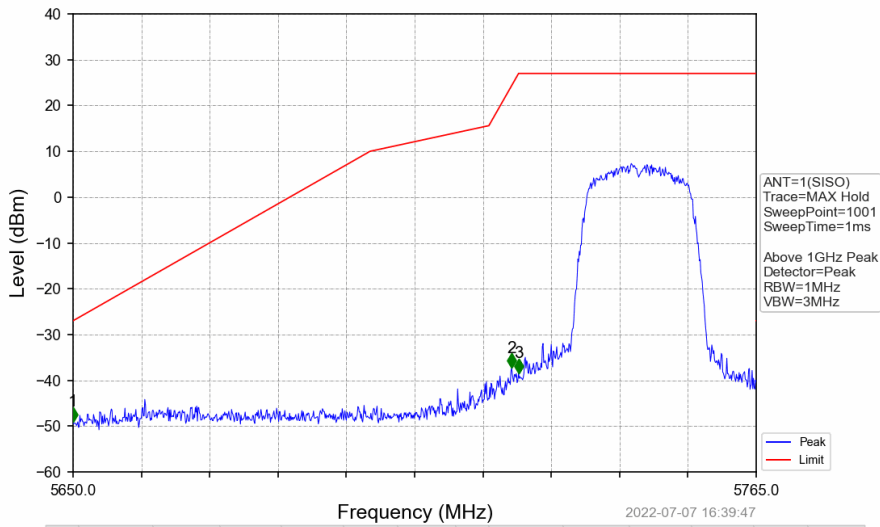
802.11n(HT20)_LCH_5745MHz_Ant1_NTNV
