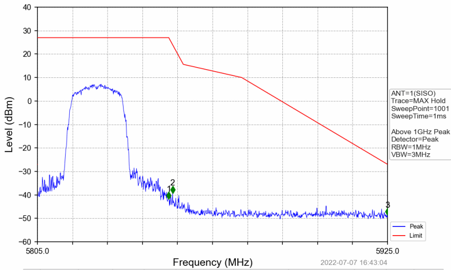
802.11n(HT20)_HCH_5825MHz_Ant1_NTNV
