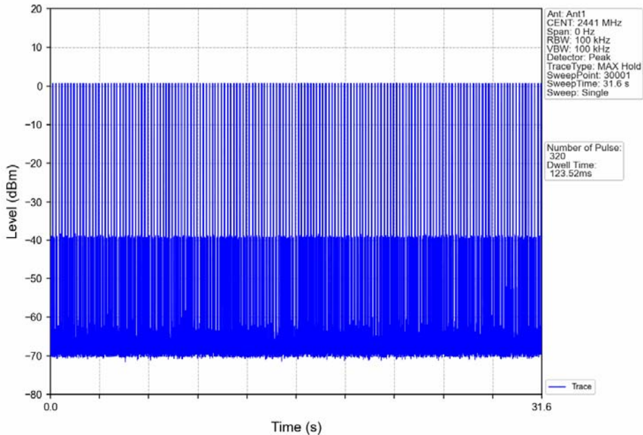
GFSK_DH1_HOPP_Ant1_NTNV
