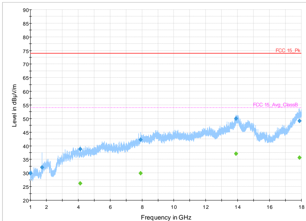
Plot 26. 1-18GHz, 1Mbps, 2480MHz
