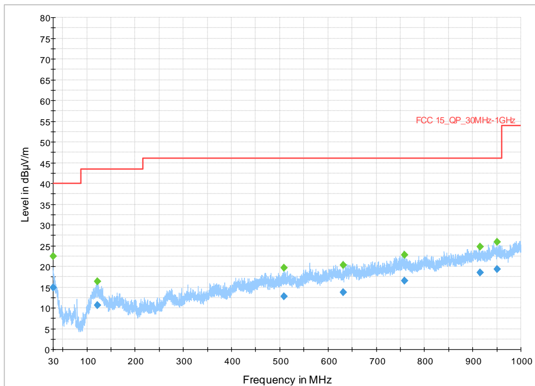
Plot 22. 30MHz-1000MHz, 1Mbps, 2440MHz
