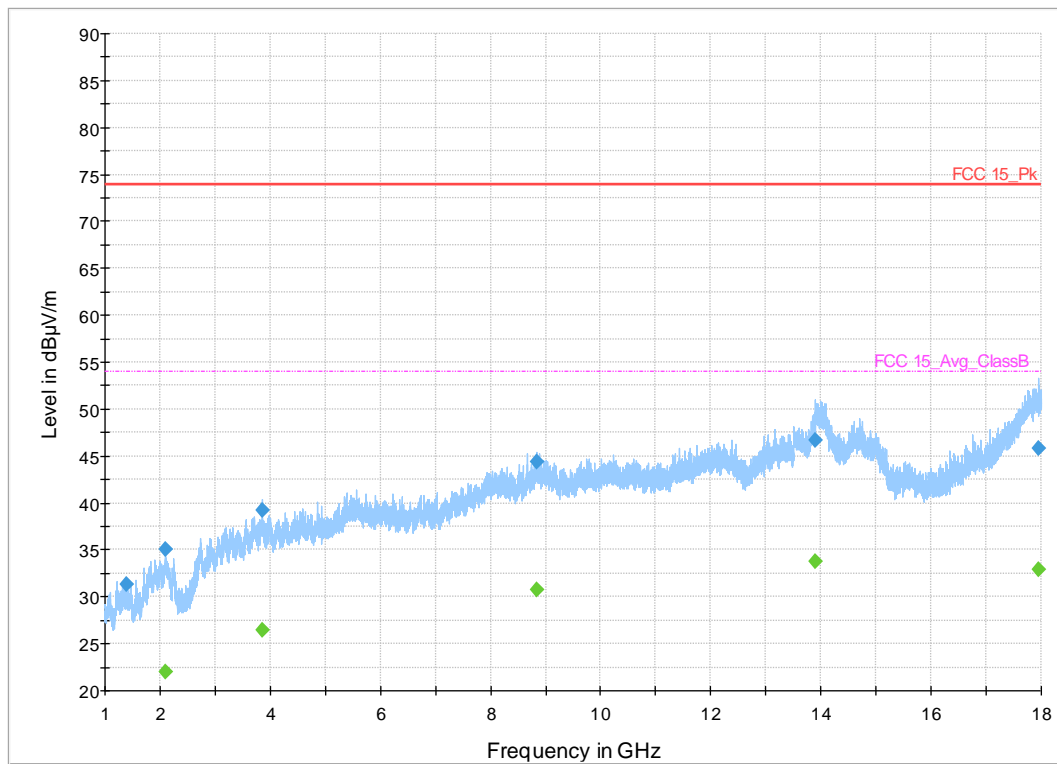
Plot 24. 1-18GHz, 1Mbps, 2402MHz
