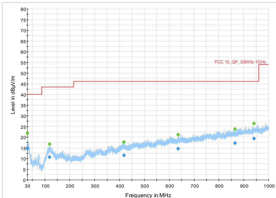
Plot 23. 30-1000MHz, 1Mbps, 2480MHz
