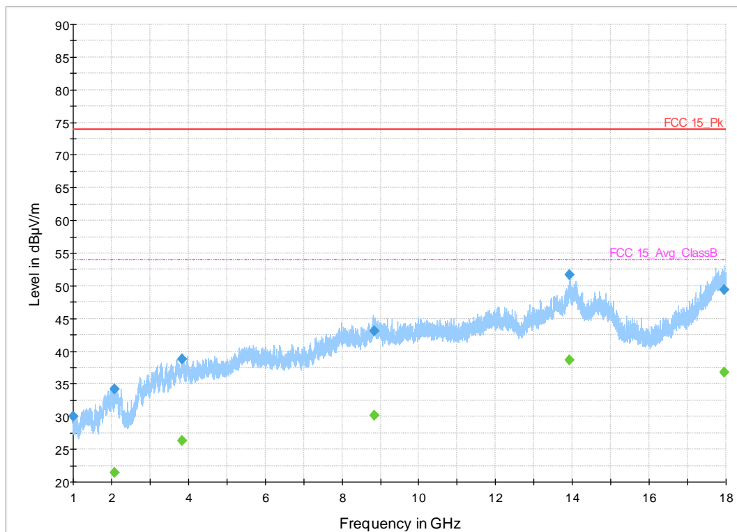
Plot 25. 1-18GHz, 1Mbps, 2440MHz
