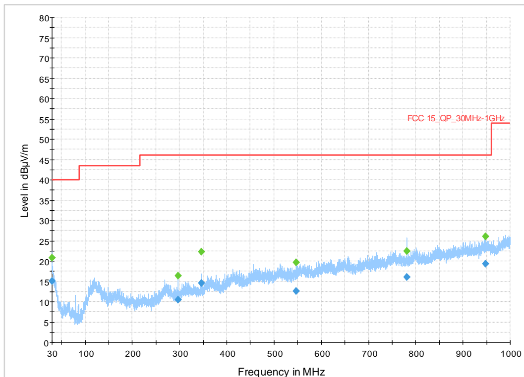
Plot 21. 30MHz-1000MHz, 1Mbps, 2402MHz
