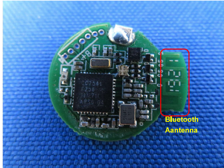
(12) EUT Photo
