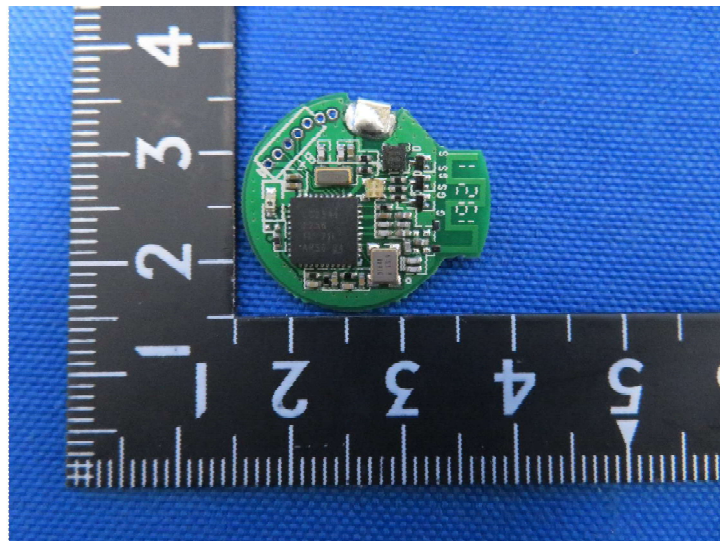
(10) EUT Photo
