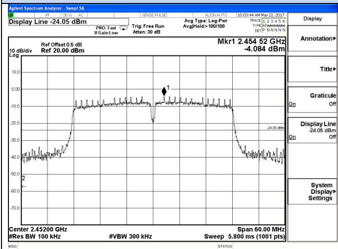
2422 – 2482 MHz
