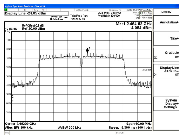
2422 – 2482 MHz
