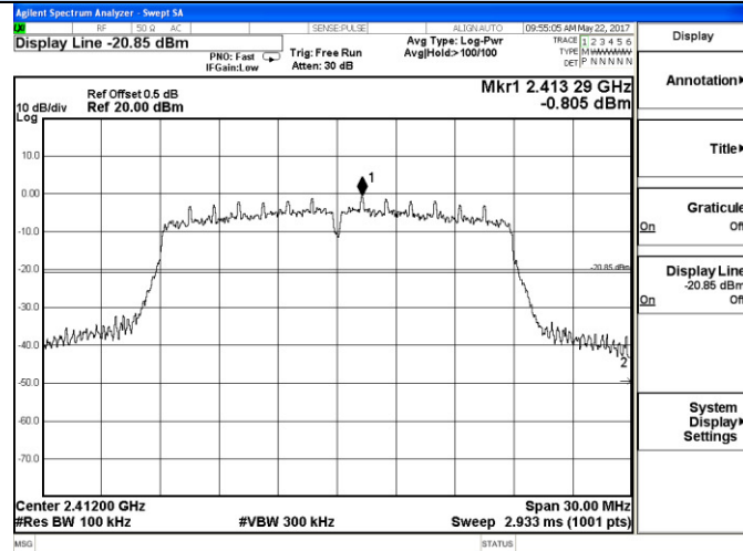
2397 – 2427 MHz
