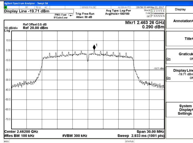
2447 – 2477 MHz
