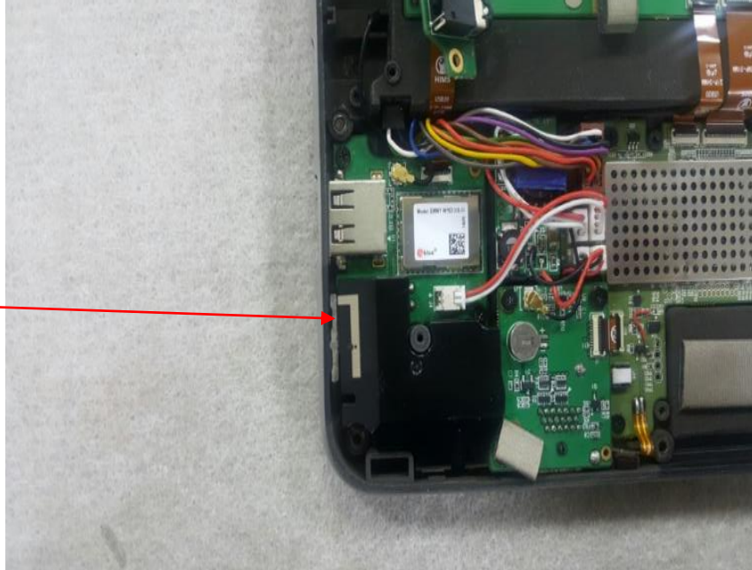
NFC ANT
