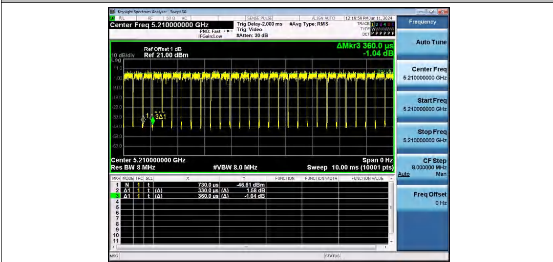
NTNV-11AC80SISO-Ant1-5210
