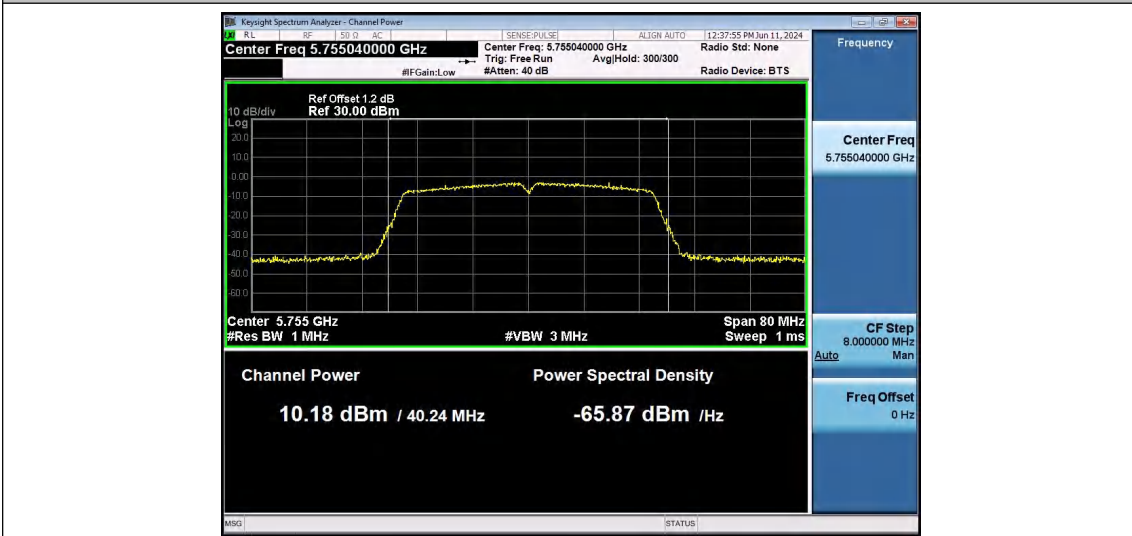
11N40SISO-Ant1-5755-PASS
