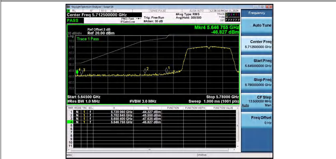
11N40SISO-Ant1-5755-PASS
