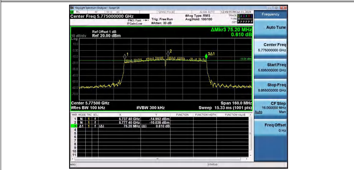
11AC80SISO-Ant1-5775-PASS
