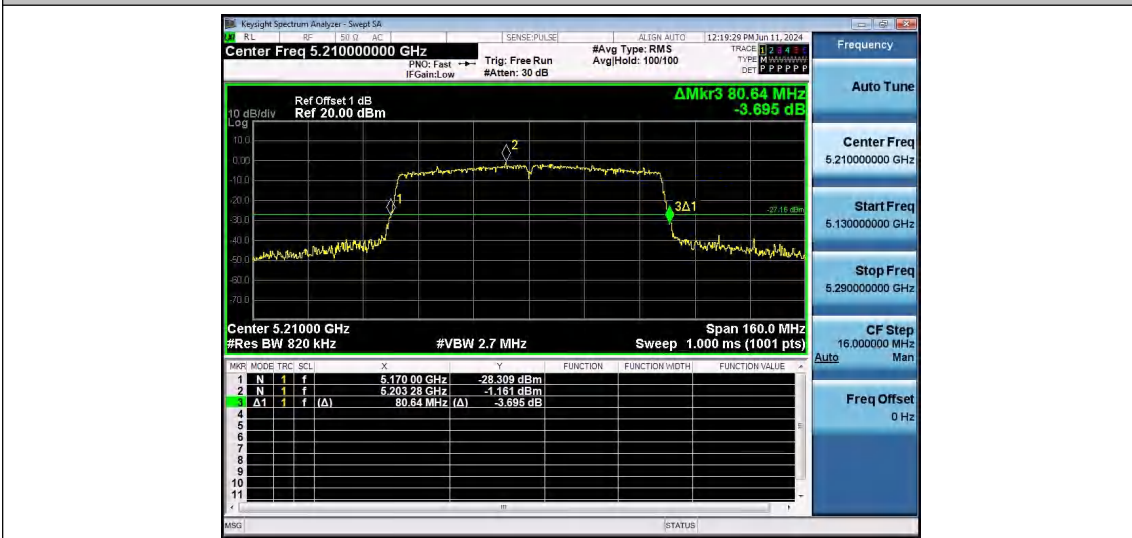
11AC80SISO-Ant1-5210
