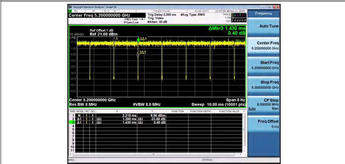
NTNV-11A-Ant1-5200
