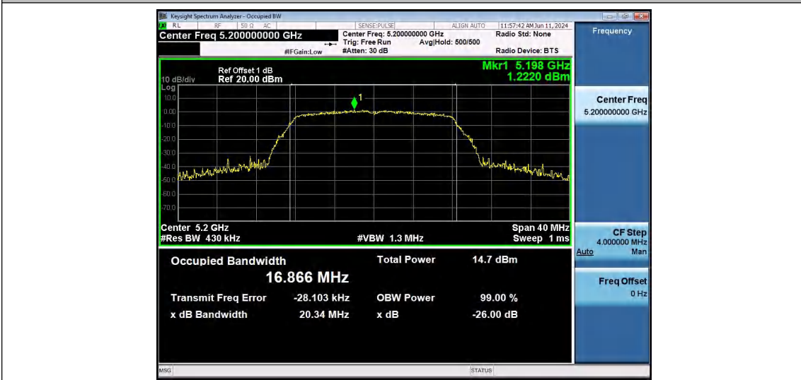
11A-Ant1-5200
