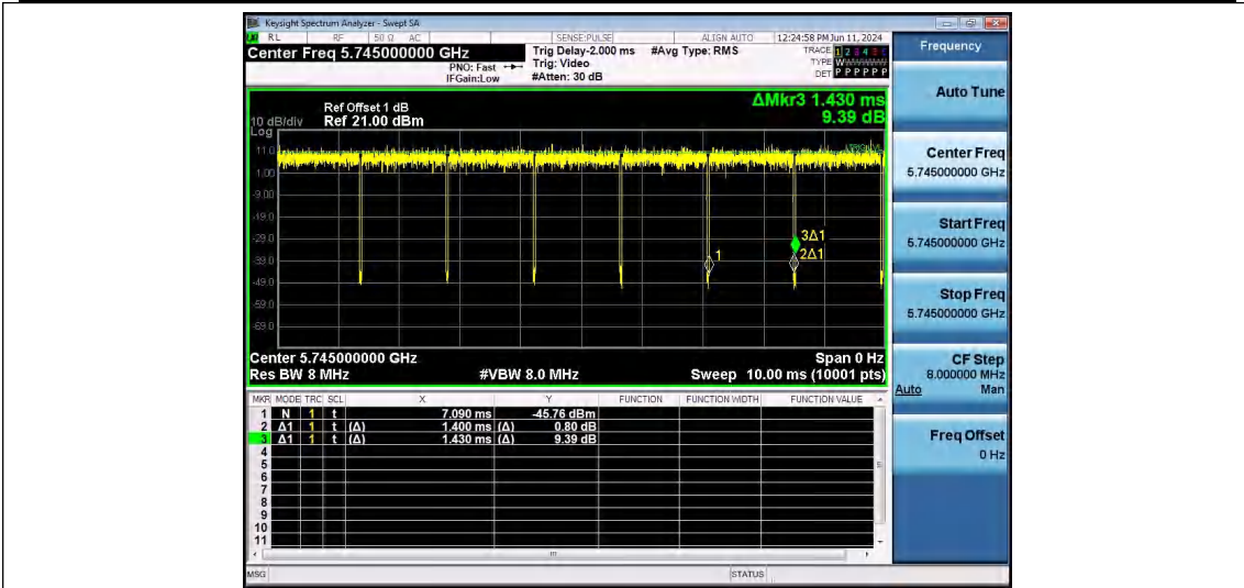
NTNV-11A-Ant1-5745
