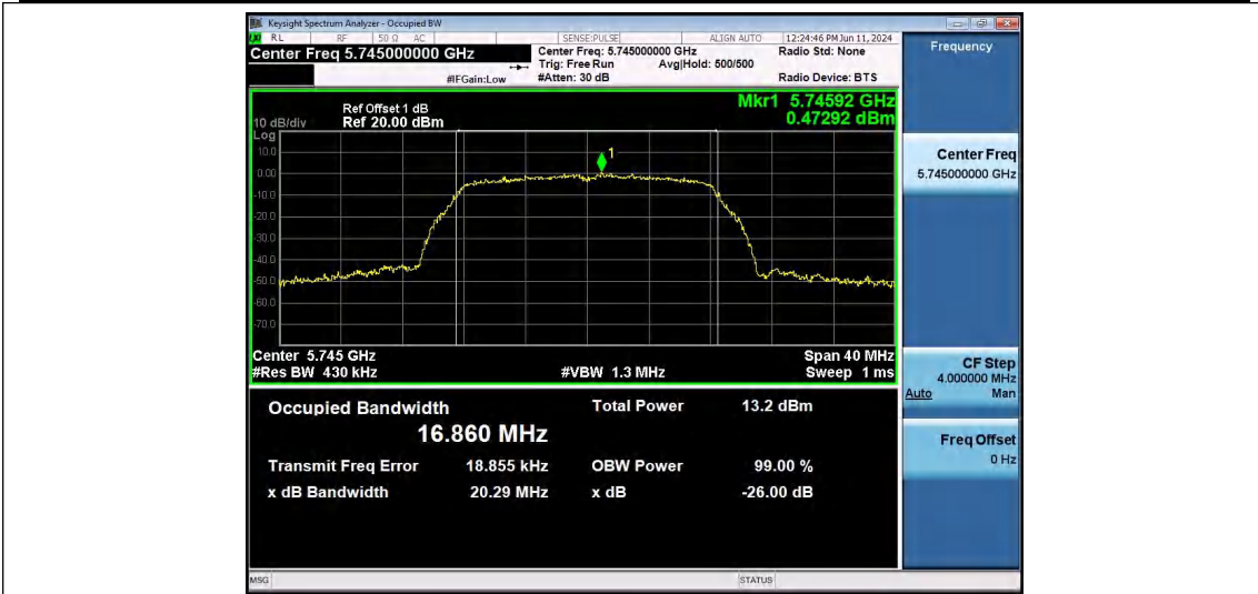
11A-Ant1-5745
