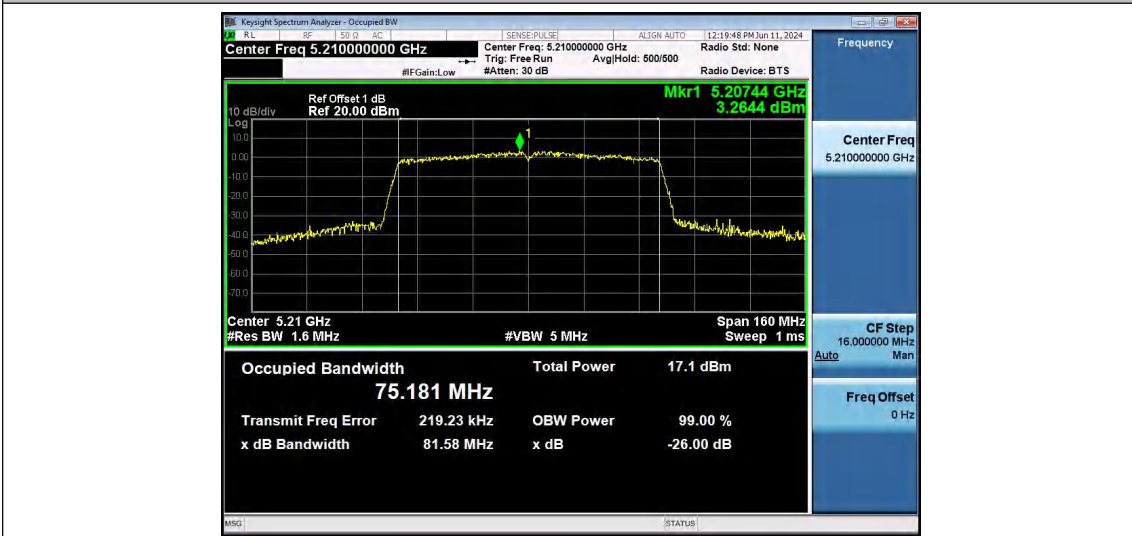
11AC80SISO-Ant1-5210
