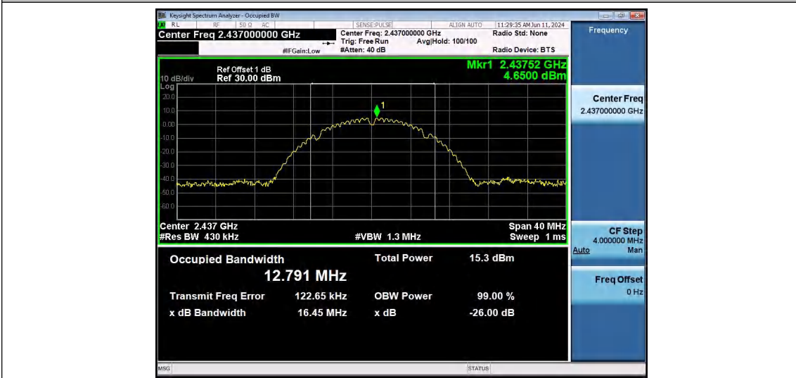
11B-Ant1-2437
