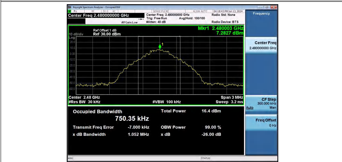
DH5-Ant1-2480
