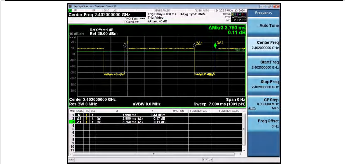
NTNV-2DH5-Ant1-2402
