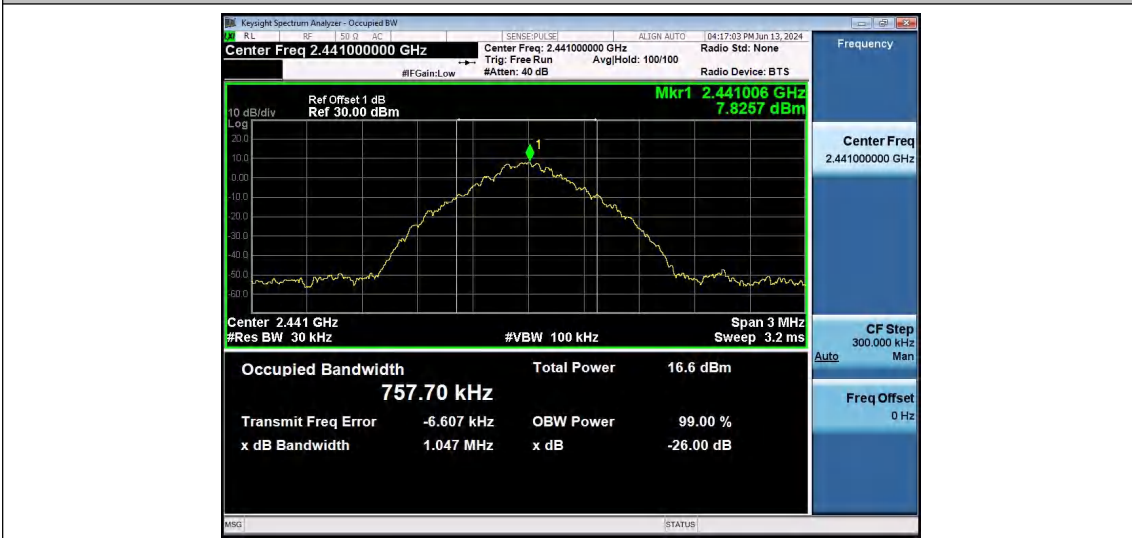
DH5-Ant1-2441
