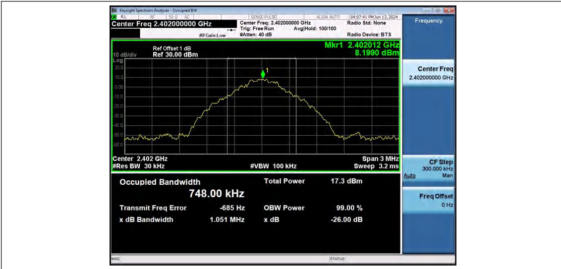
DH5-Ant1-2402
