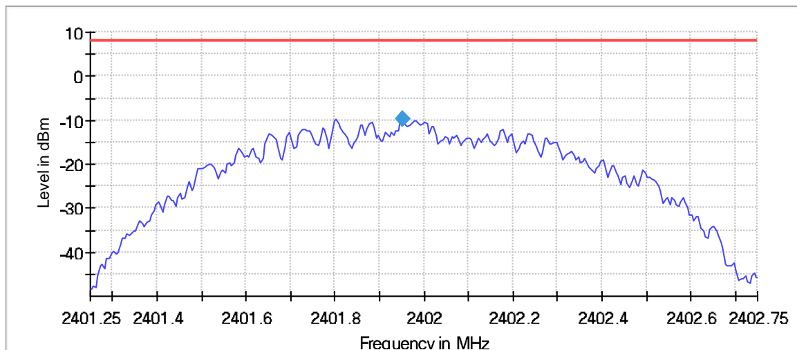
Power Spectral Densitiv (AVGPSD-3)
