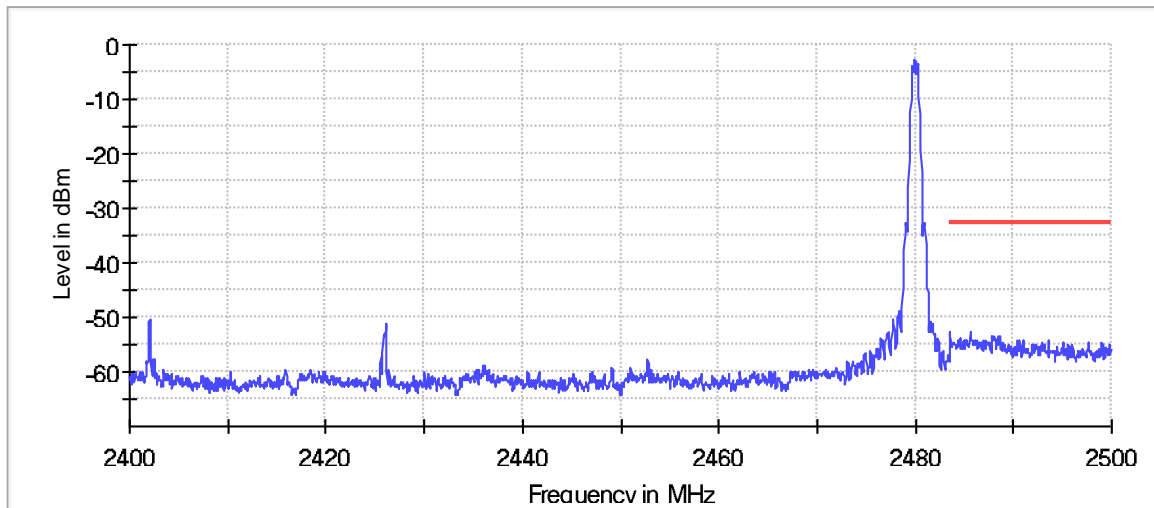
Band Edge
