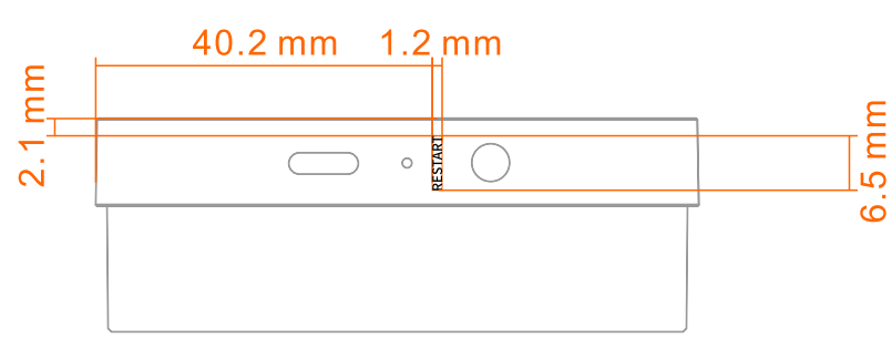
底面
