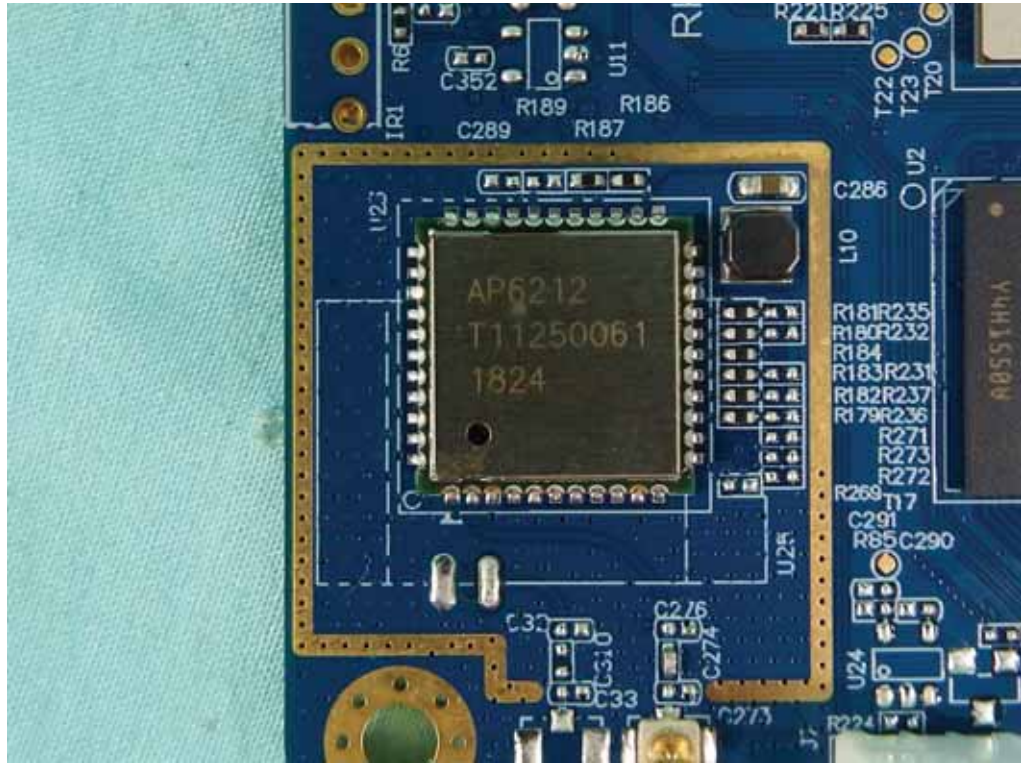
RF module
