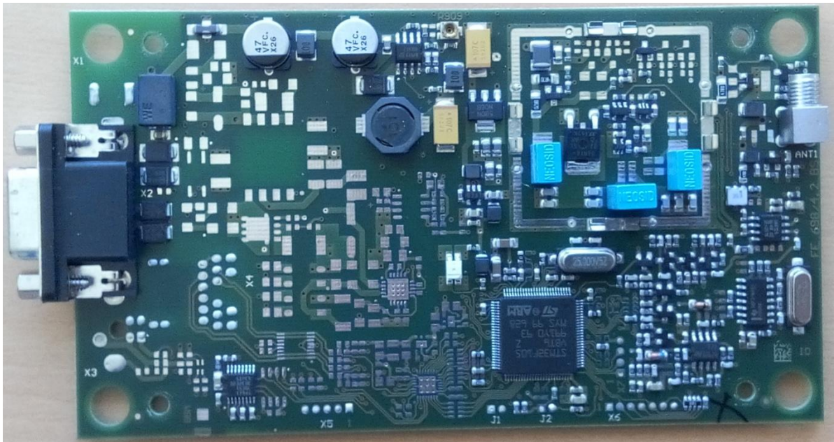
ID ISC.MRM102-A Top without plating
