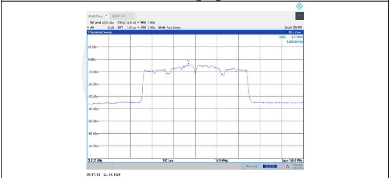
11AC80SISO_Ant1_5210
