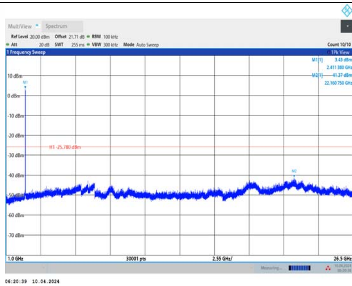
11B_Ant1_2437_0~Reference
