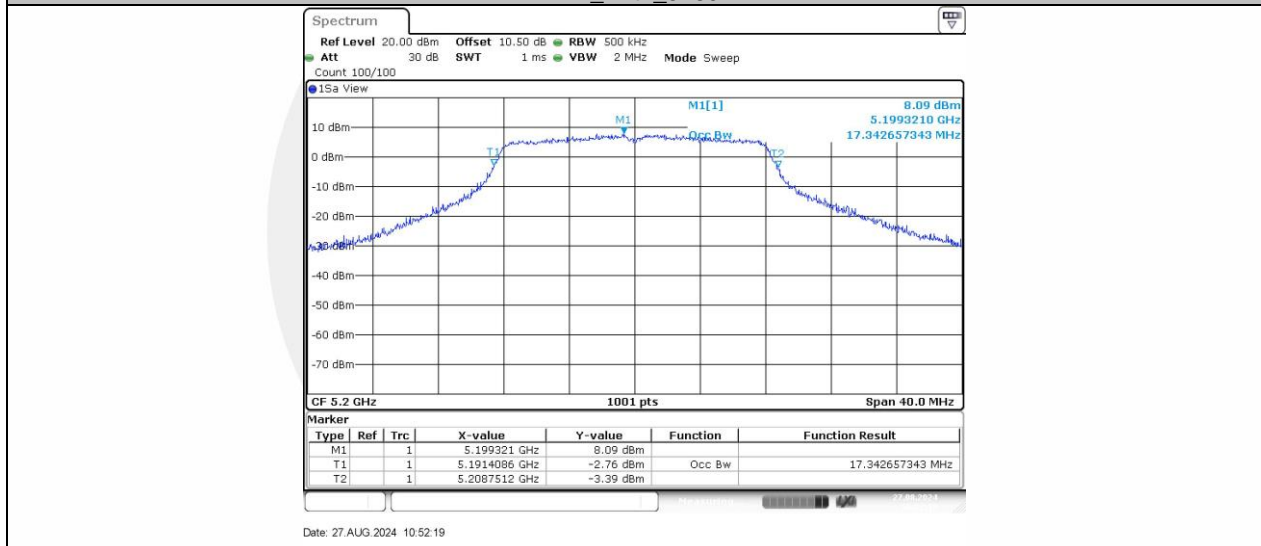
11A_Ant1_5200
