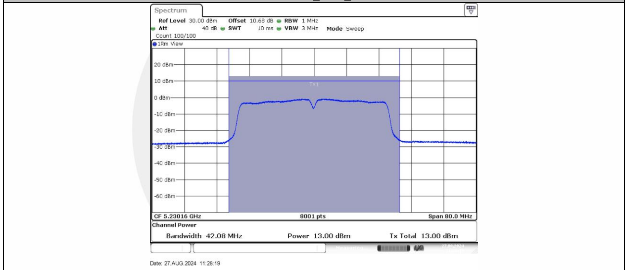
11N40SISO_Ant1_5230
