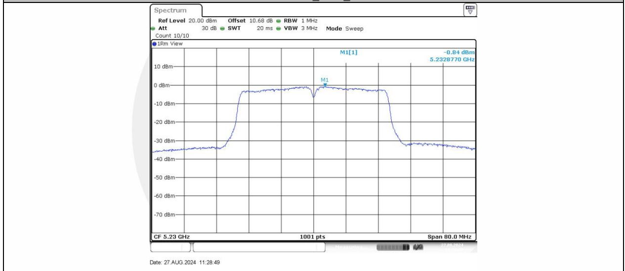
11N40SISO_Ant1_5230
