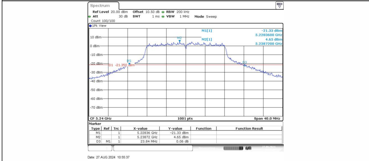
11A_Ant1_5240
