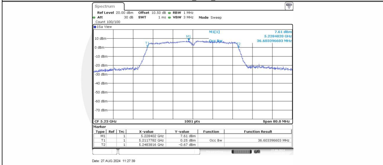
11N40SISO_Ant1_5230
