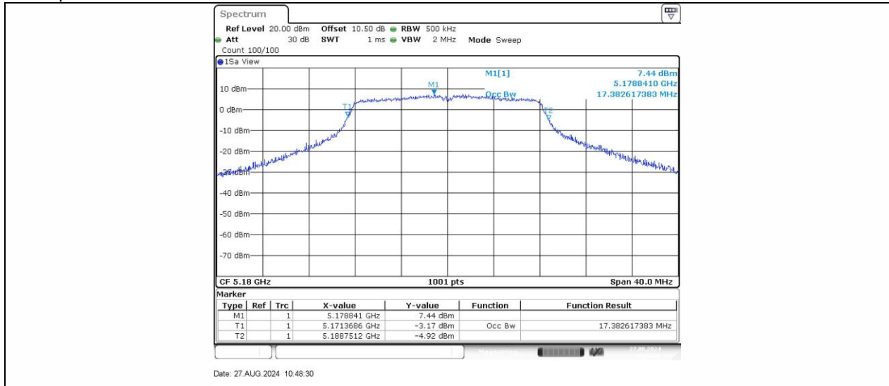
11A_Ant1_5180
