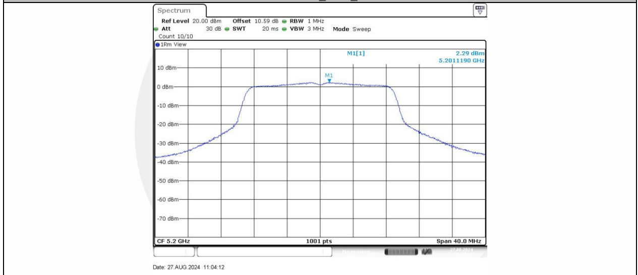
11N20SISO_Ant1_5200
