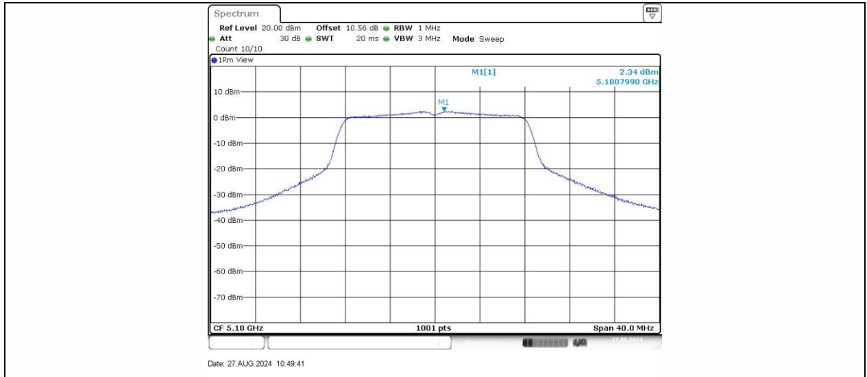
11A_Ant1_5180
