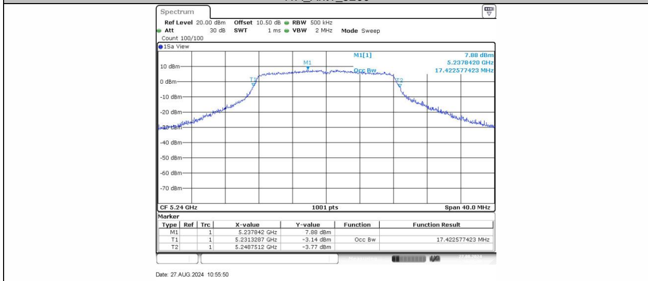
11A_Ant1_5240
