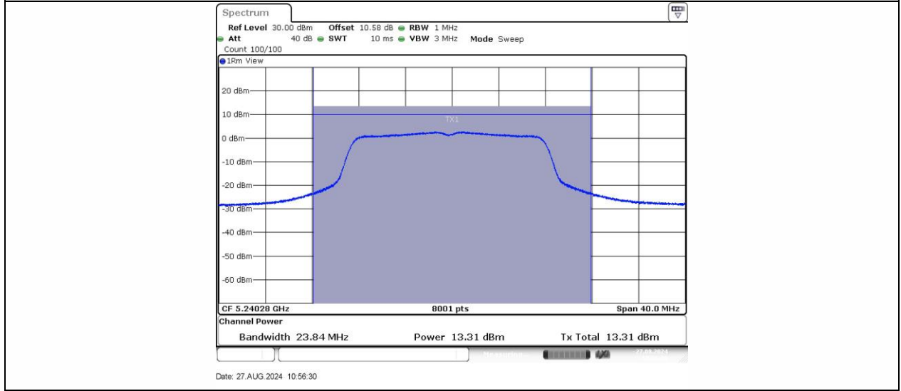
11A_Ant1_5240
