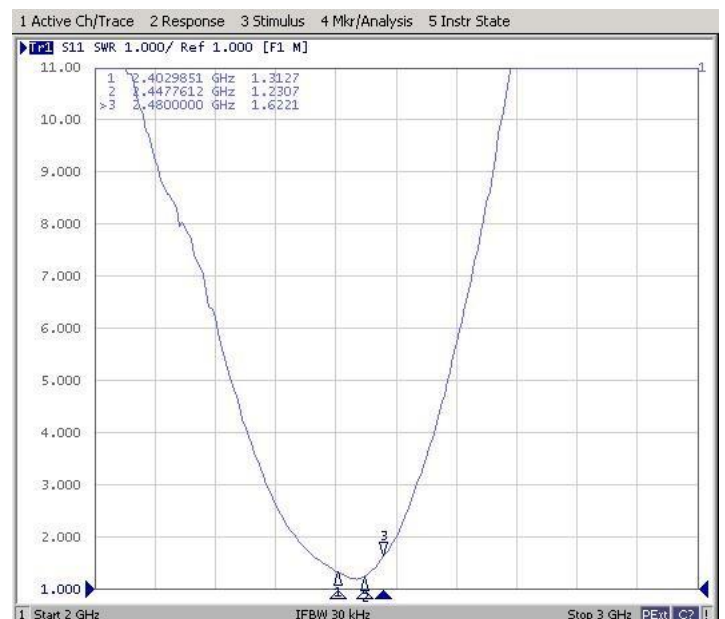
VSWR
