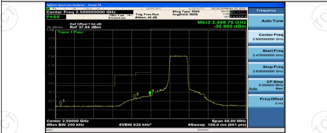
Band7-10MHz-QPSK-20800-25RB#0
