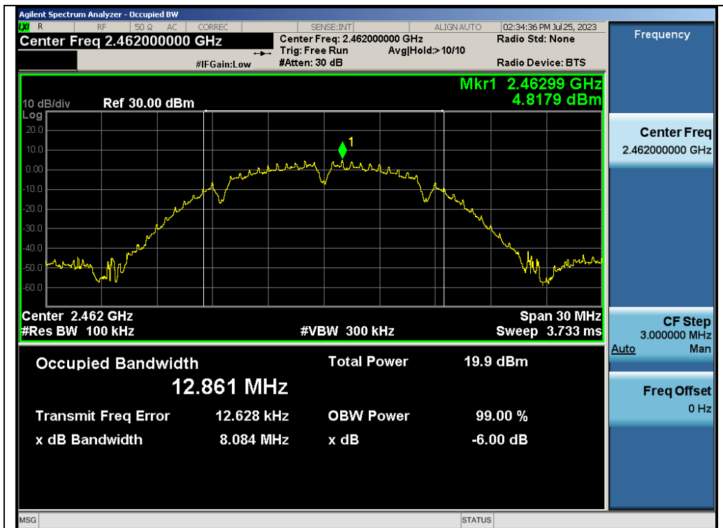
Test_Graph_802.11b_ANT1_2462_1Mbps_DTSBW
