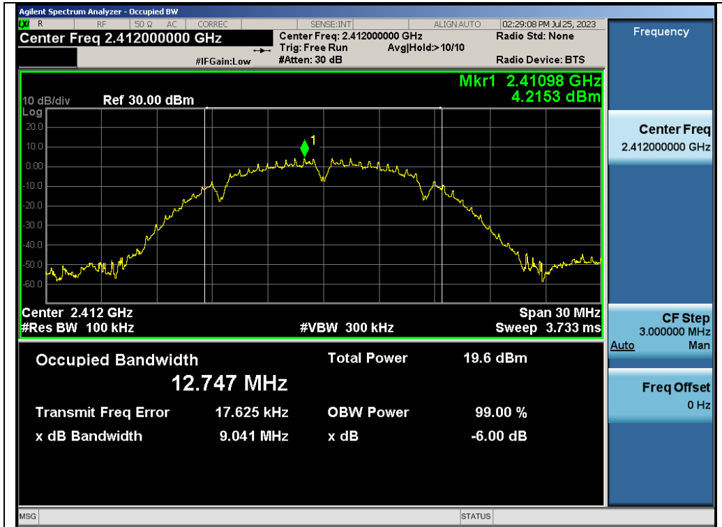
Test_Graph_802.11b_ANT1_2412_1Mbps_DTSBW
