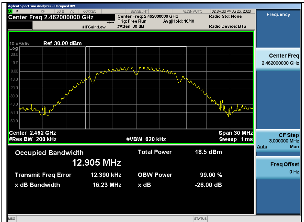
Test_Graph_802.11b_ANT1_2462_1Mbps_OBW
