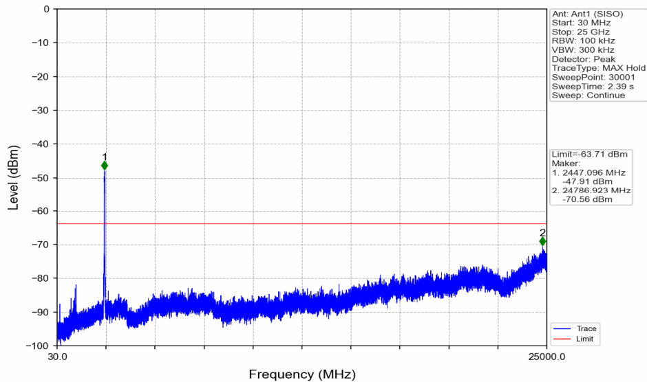
802.11n(HT40)_HCH_2452MHz_Ant1 (SISO)_NTNV
