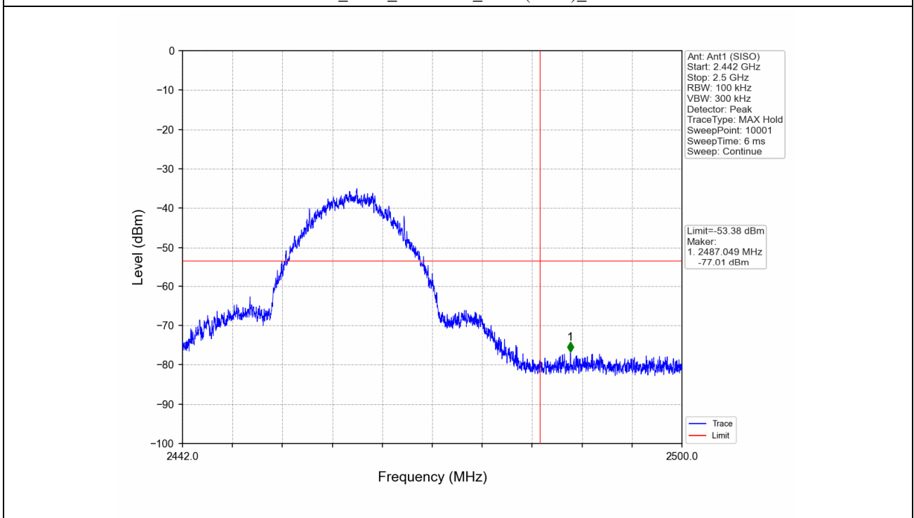
802.11b_HCH_2462MHz_Ant1 (SISO)_NTNV
