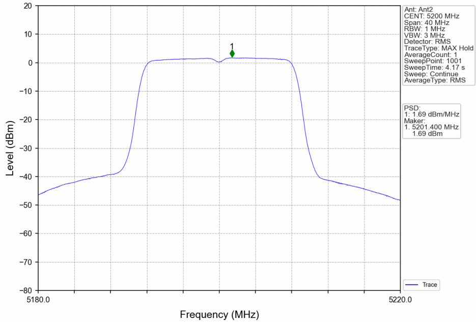
802.11n(HT20)_MCH_5200MHz_MIMO_NTNV
