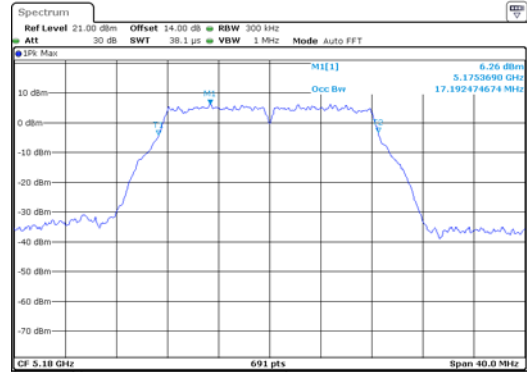
ANT 2(11A)
