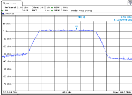
ANT 1(11AC20)
