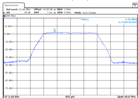
ANT 2(11A)
