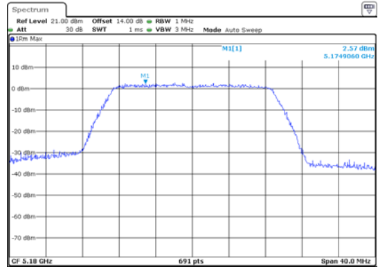
ANT 2(11AC20)
