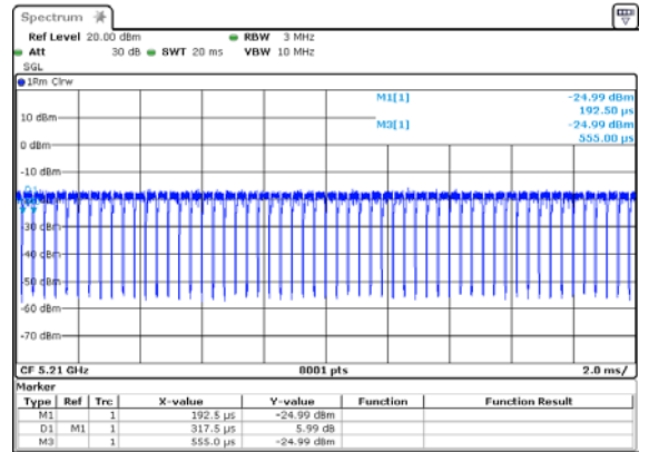
ANT 2
