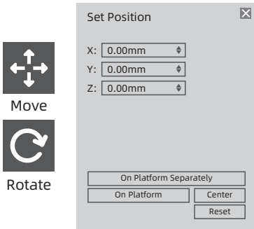
FlashDental.exe
