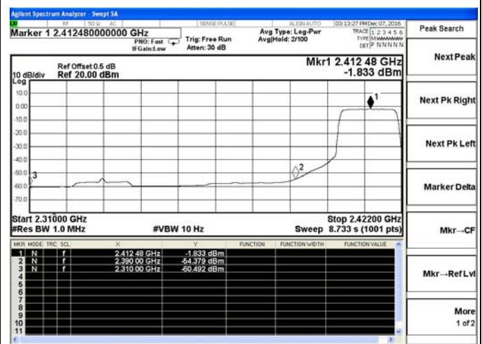
802.11g-Low channel(Average)
