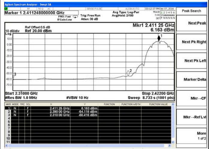
802.11b-Low channel(Average)
