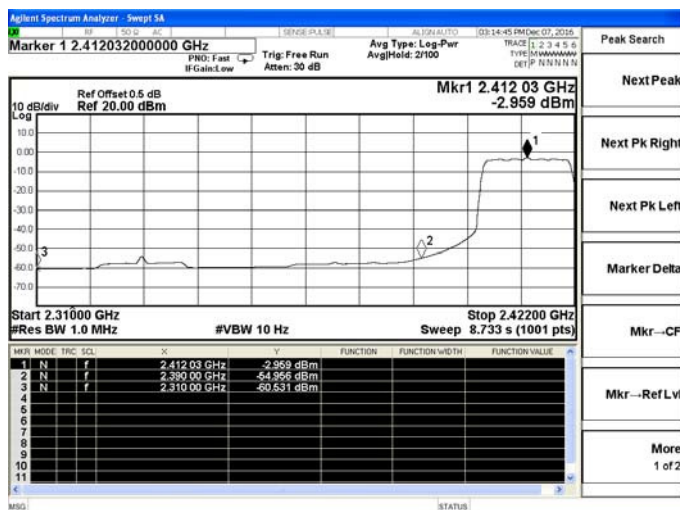
802.11n(HT20)-Low channel(Average)
