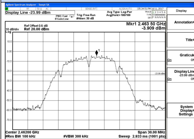
2447 – 2477 MHz
