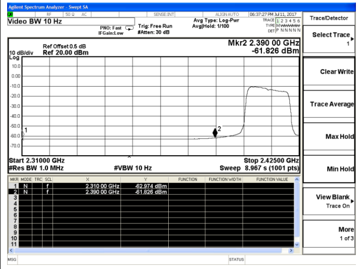
802.11g Low channel(Average)
