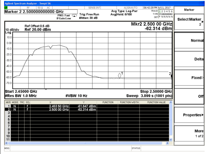
802.11b High channel(Average)
