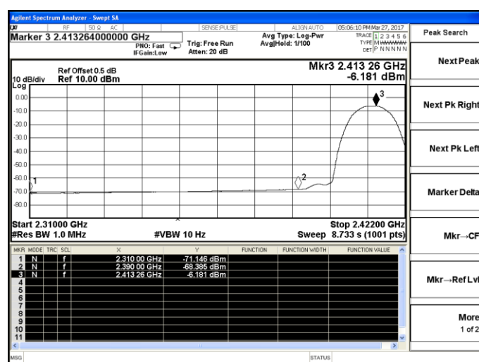
802.11b-Low channel(Average)
