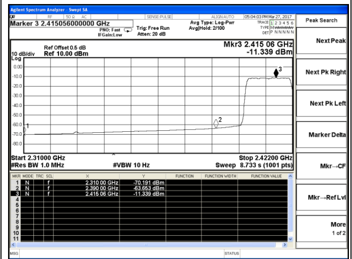
802.11n-HT20-Low channel(Average)
