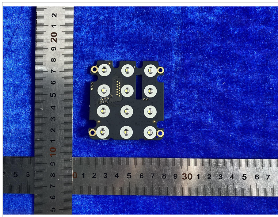
EUT-12
